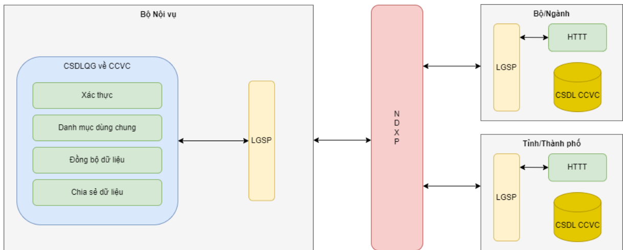
Mô hình dữ liệu
